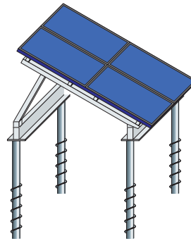
太陽光発電設備
